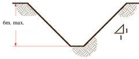
TALUD SIMPLE TIPO DE SUELO B
